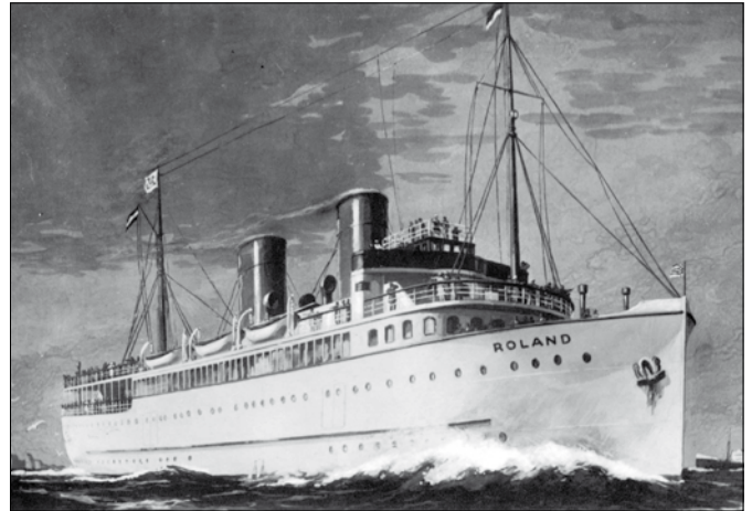
Abb. 1: Turbinendampfer „Roland“ des NDL. Bauwerft: Deutsche Schiffs- und Maschinenbau AG, Werk Tecklenburg Bremerhaven. Stapellauf am 12. März 1927. 18 Knoten. 2 400 Passagiere. 1
